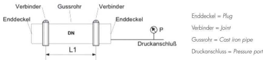
Bild 2-2: Prüfaufbau „Unterdruckprüfung der Verbindungen“ von DN 50 bis DN 300
