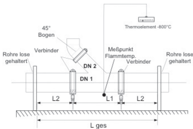
Bild 2-3: Prüfaufbau „Flammprüfung der Verbindungen“ von DN 50 bis DN 150
