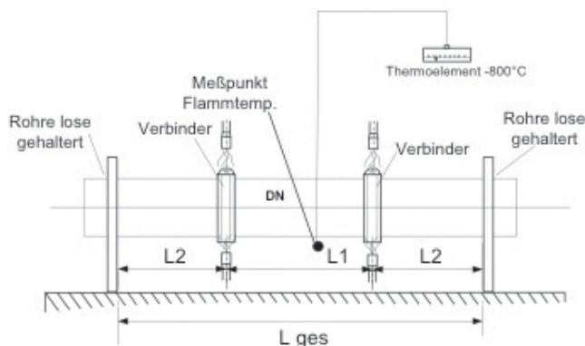
Bild 2-4: Prüfaufbau „Flammprüfung der Verbindungen“ von DN 200 bis DN 300
